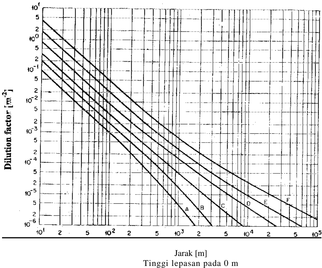
GAMBAR. E1. Faktor dilusi sebagai fungsi jarak arah angin.
