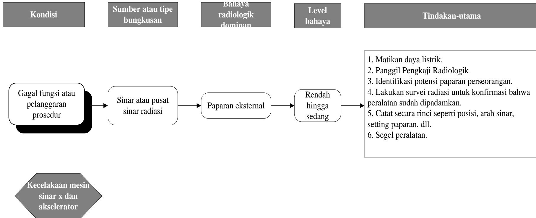
Gambar B7: Mesin Sinar -X dan akselerator
